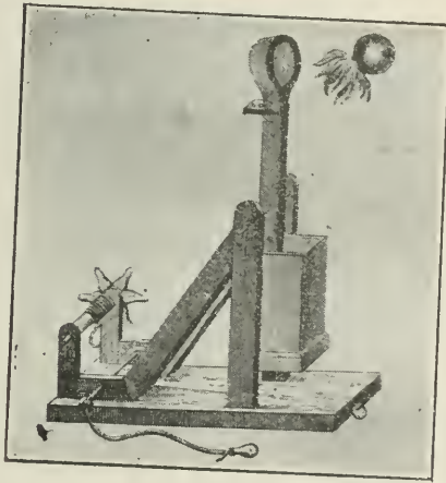
ش ٤٤ : آلة رمي قارورة النفط مشتعلة للاحراق
